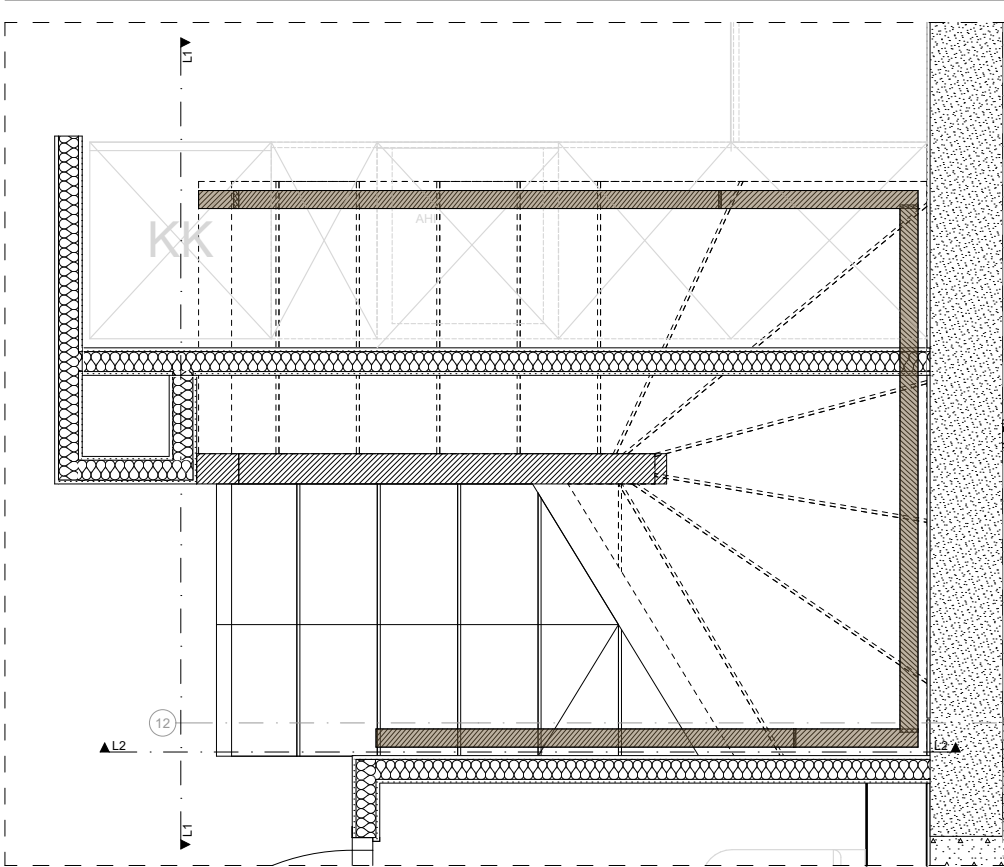
PEALTVAADE 1k
