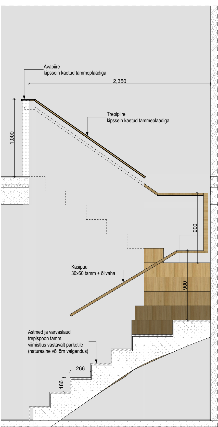
TREPI LÕIGE 2
