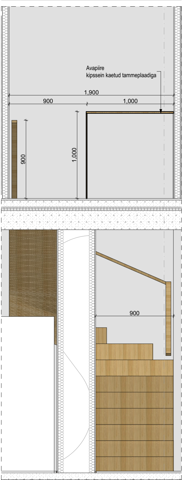
TREPI LÕIGE 1
